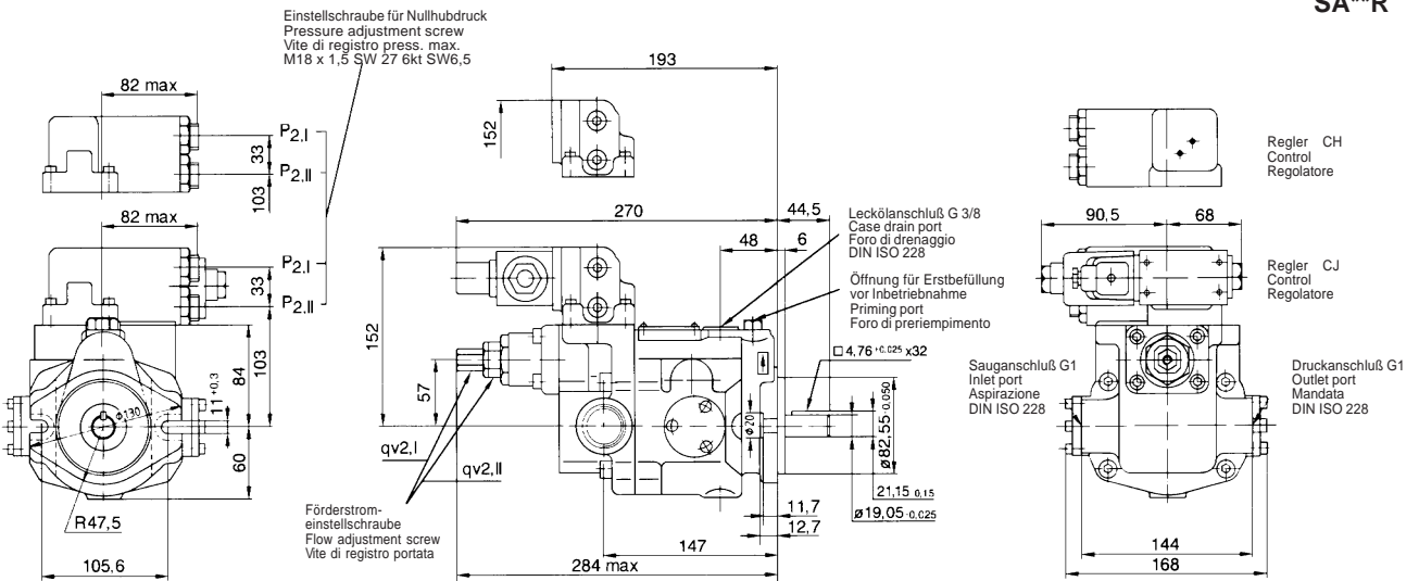
Bild / Fig. 38: Baugröße · Model · Grandezza J-V15C**RHx C**RJ*X
