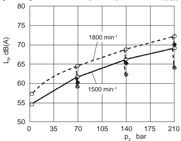
Bild / Fig. 6: Baugröße · Model · Grandezza J-V 15
